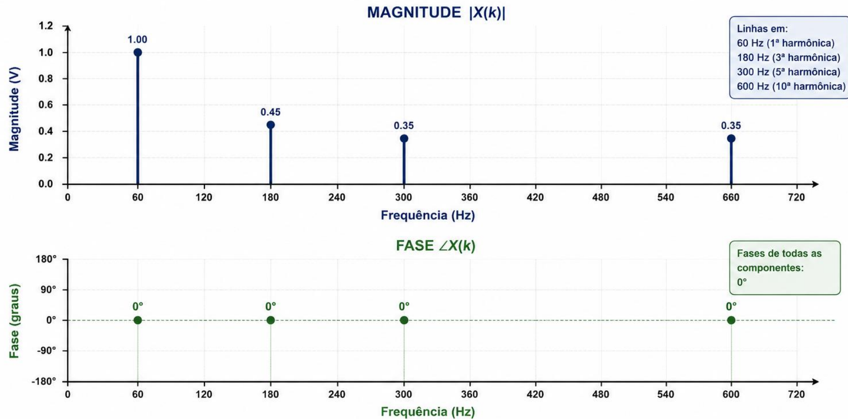
Resumo das Componentes Espectrais
